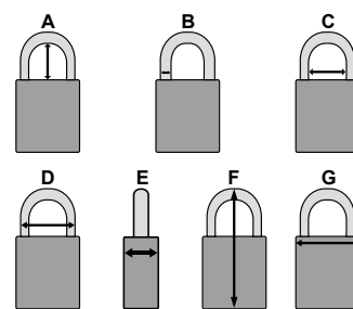
【サイズ】 A : 38mm、B : φ6.5mm、C : 20mm、 D : 33mm、E : 19.5mm、F : 86.5mm、 G : 38mm
