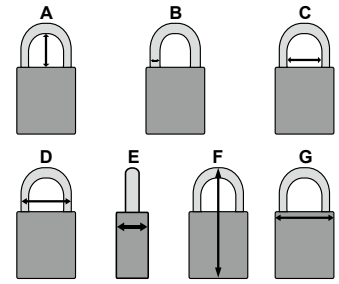
【サイズ】 A : 38mm, B : φ6.5mm, C : 20mm, D : 33mm, E : 19.5mm, F : 122mm, G : 38mm
