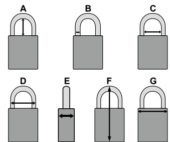
【サイズ】 A : 106.68mm / 203.2mm, B : φ4.7mm, C : 17mm, D : 26mm, E : 16mm F : -, G : 32mm
