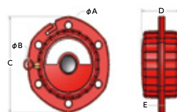
【サイズ】 A:7.75mm、B:1.7mm、C:100.8mm、 D:45.27mm、E:7.62mm
