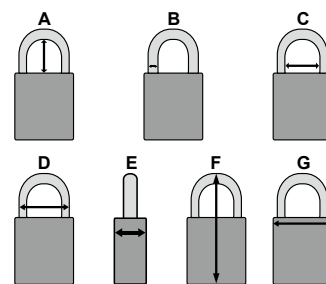
【サイズ】 A : 38mm、B : φ6.5mm、C : 20mm、 D : 33mm、E : 19.5mm、F : 86.5mm、 G : 38.5mm
