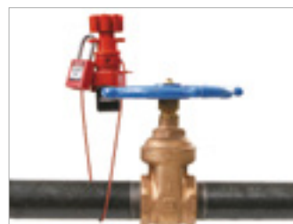
ケーブルでゲートバルブをロック。
